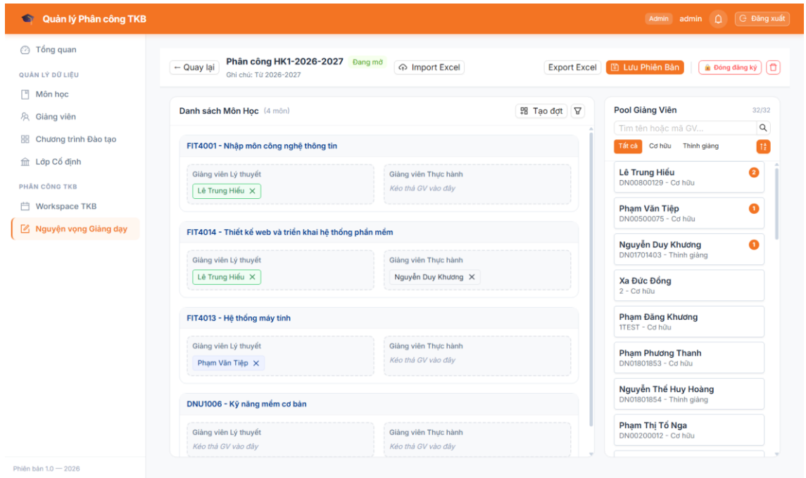
Hình Error! No text of specified style in document..8 Giao diện trang xem chi tiết đợt đăng ký nguyện vọng giảng dạy
